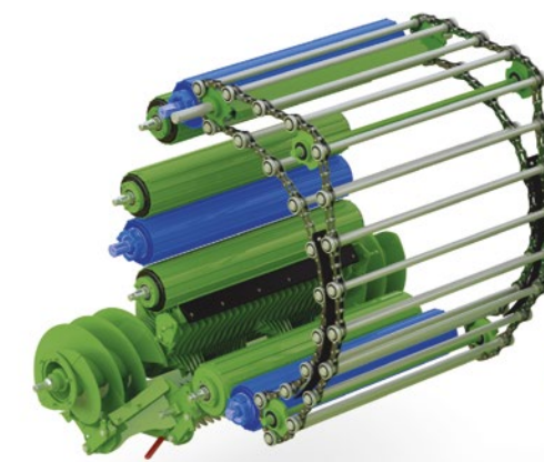
Sistem cu conveyer Multi-crop
